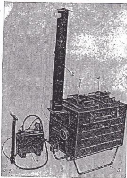
Рис. Кухня переносная МК-30: 1 — тепловой блок; 2 — дымовая труба; 3 — котел для первого блюда; 4 — котел для второго блюда; 5 — са- лазки; 6 — вентиль форсунок; 7 — топливный бак; 8 — топливопровод; 9 — ручной насос
