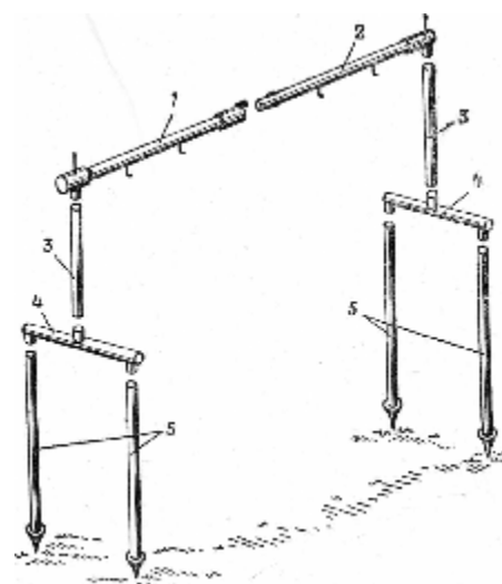
Рис. Металлический станок палатки УЗ-68
